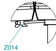
Einzelheit B
