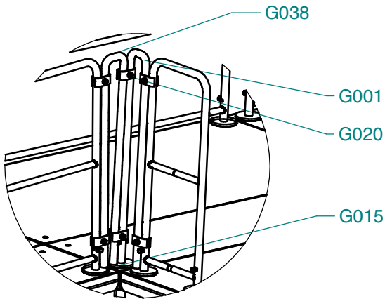
Einzelheit A
