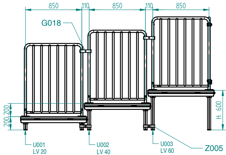
Ansicht rechts
