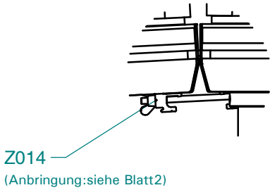
Einzelheit B
