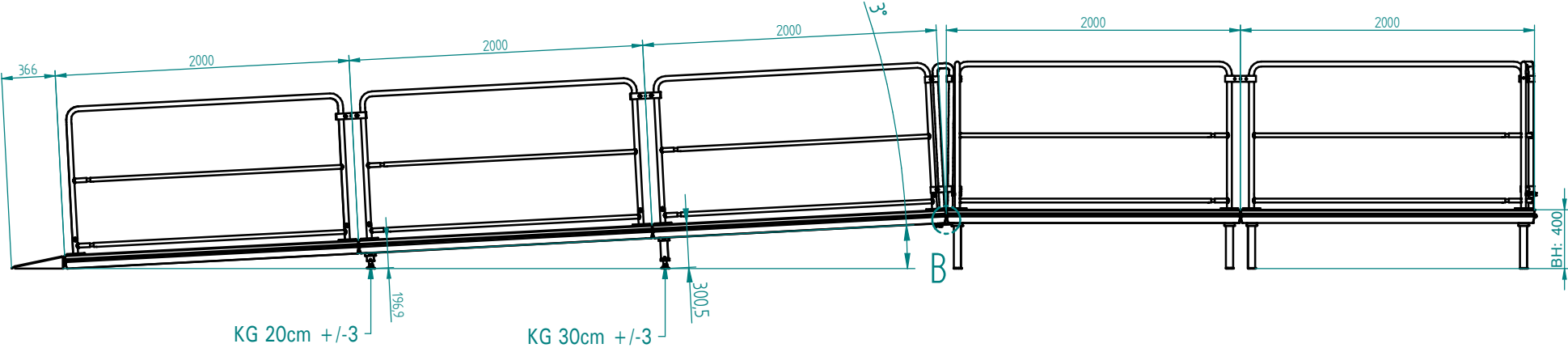
Einzelheit B
